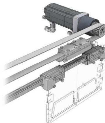
D'entraînement avec servomoteur, réducteur planétaire, courroie dentée et guidage à bille
